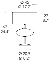
LSH07 E27 ELLISSE / ELLIPSE
