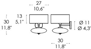
LSH23 E27 ELLISSE / ELLIPSE
