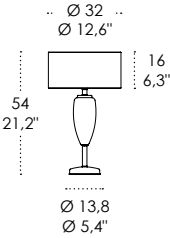
LSH02 E27 OGIVA / OGIVE
