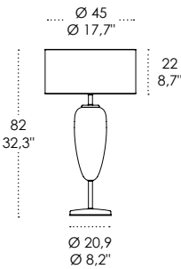
LSH06 E27 OGIVA / OGIVE
