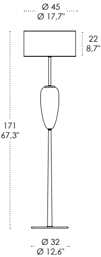
LSH12 E27 OGIVA / OGIVE
