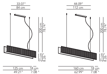
Pendant lamp
