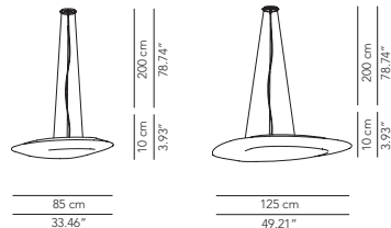
Pendant lamp
