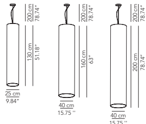
Pendant lamp
