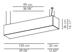
Pendant lamp
